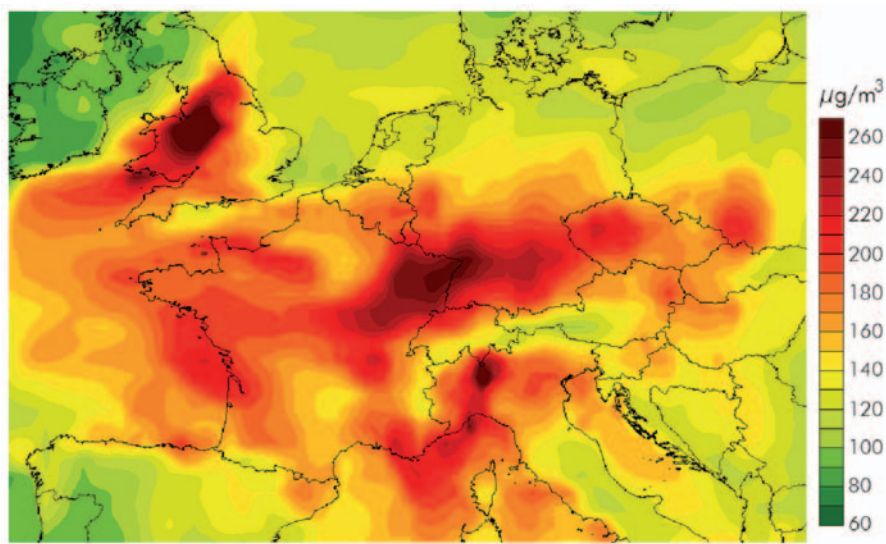
Image 1 : maxima d'O 3 , le 4 août 2003 sur l'Europe centrale (en \mu\text{g}/\text{m}^3 simulé par le Laboratoire interuniversitaire des systèmes atmosphérique (LISA)
