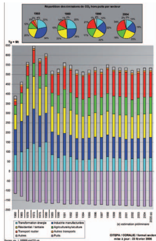
Graphique 4 : émission de CO 2 dans l'air en France métropolitaine
