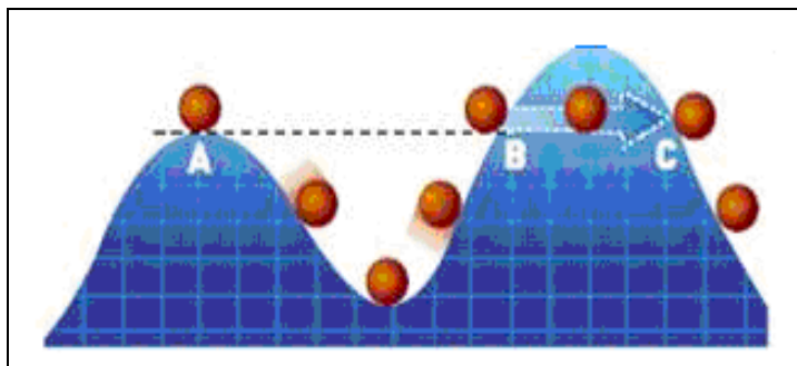
Schéma 3 : Un exemple d'effet à l'échelle nanométrique : l'effet tunnel
