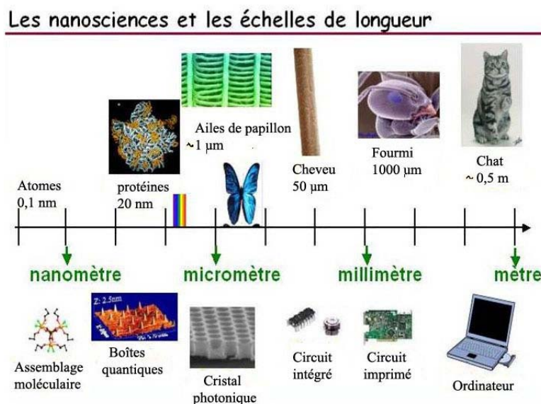
Schéma 1 : Les nanosciences et les échelles de longueur
