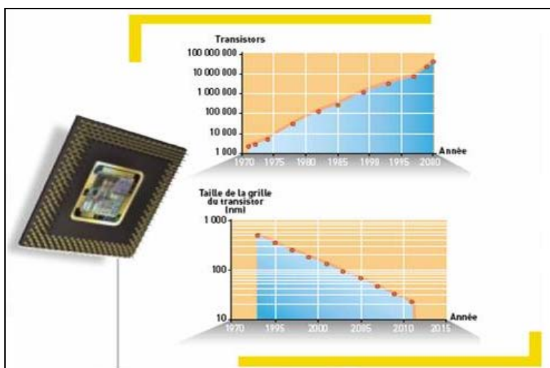
Schéma 8 : Taille et nombre de transistors dans un circuit intégré
