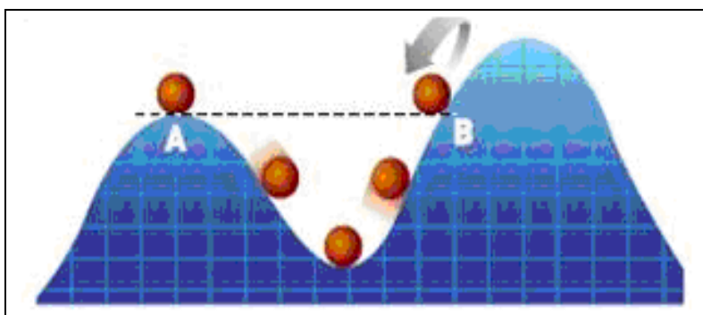
Schéma 2 : Un exemple d'effet à l'échelle macroscopique
