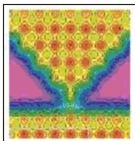
Schéma 5 : Pointe de microscope effet tunnel à proximité d'une surface simulée par ordinateur
