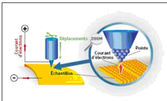
Schéma 5 : Pointe de microscope effet tunnel à proximité d'une surface simulée par ordinateur
